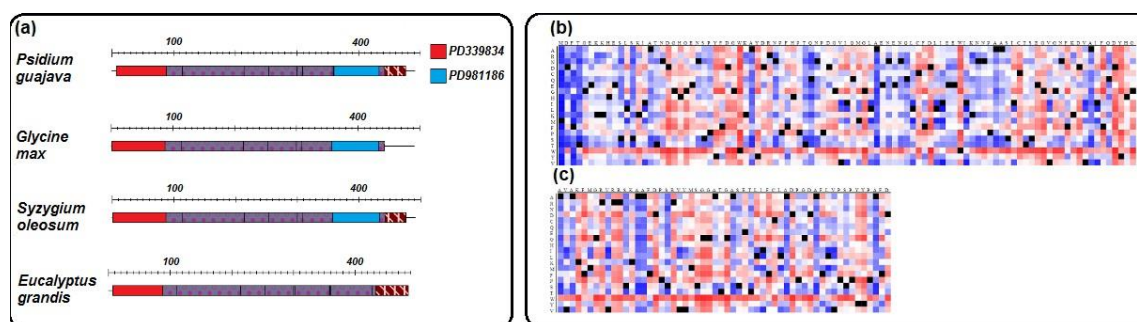
Figura2. Previsão dos efeitos funcionais das mutações em aminoácidos pelo servidor SNAP2 e Domínios funcionais da 1-aminociclopropano-1-carboxilato sintase observados pelo servidor ProDom.
