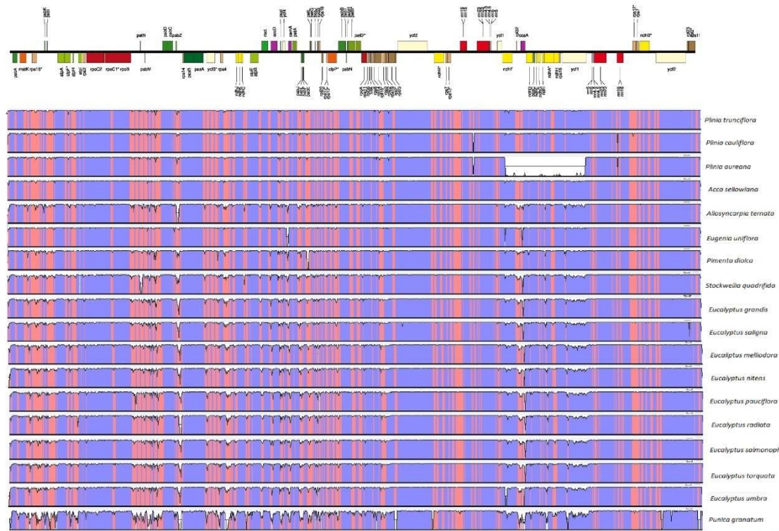
Figura 1. Alinhamento de sequências completas de plastomas de 18 espécies da família Myrtaceae. Regiões em azul identificam regiões codificantes segundo anotação para P. guajava , obtida pelo servidor DOGMA. A representação linear do Plastoma de P. guajava foi obtida pelo servidor OGDRAW (Lohse et al., 2013). Regiões em rosa representam regiões não-codificantes conservadas. A espécie P. granatum foi utilizada como grupo externo, representando a família Lythraceae. SV = Sítios variáveis.
